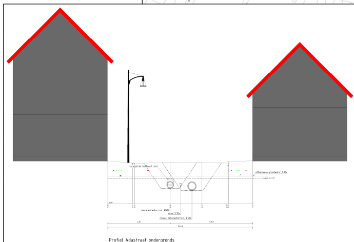
PROFIEL INCL. ONDERGRONDSE INFRA
